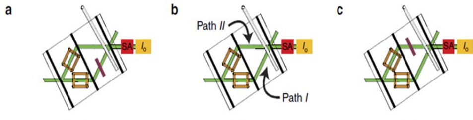
Denkmayr et al. Figure 3 Absorber
